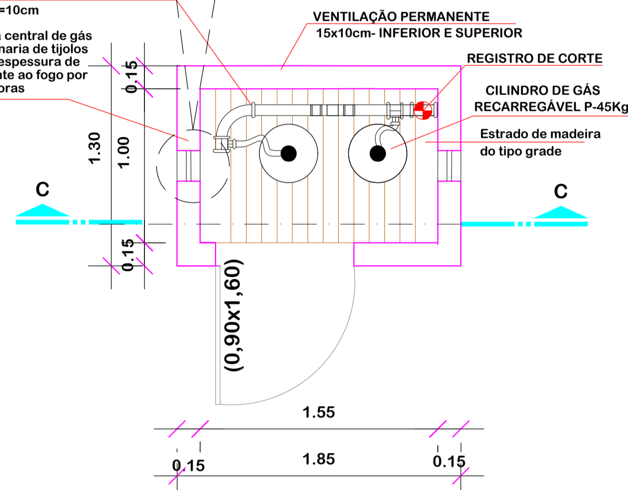
PLANTA BAIXA- CENTRAL DE GÁS ESC:1/25
