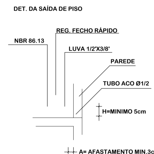
DET. DA SAÍDA DE PISO
