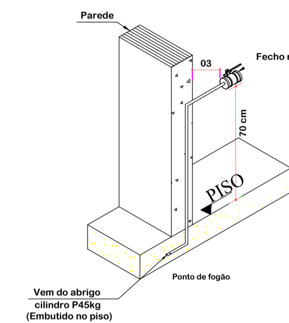
DETALHE REGISTRO DE CORTE ESC.:SEM ESCALA
